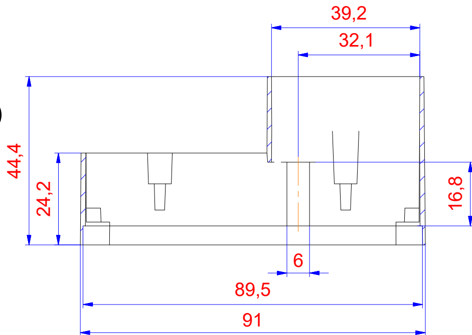
C-C ( 1 : 1 )
