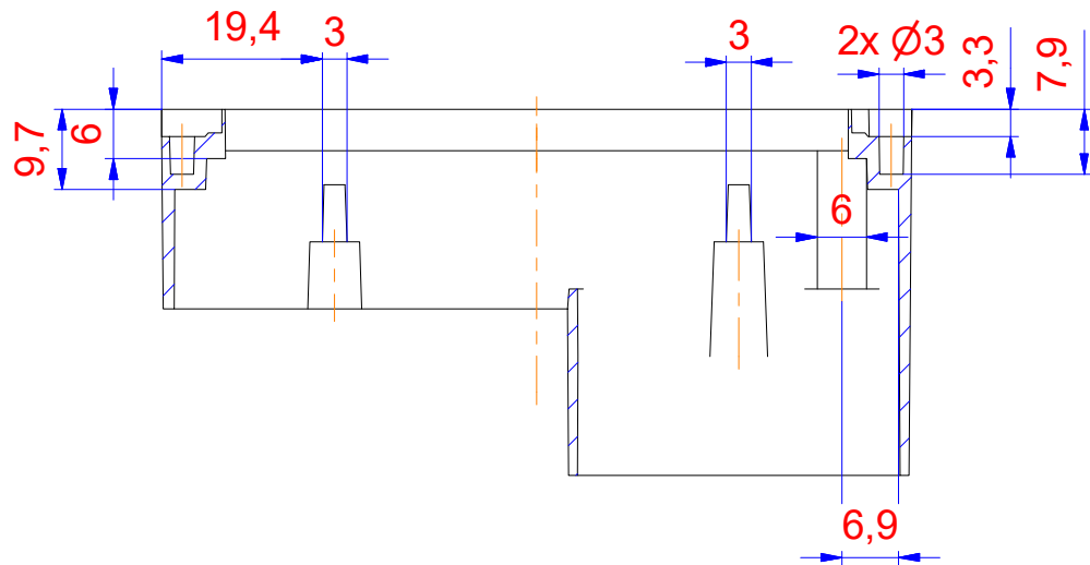
A-A ( 1 : 1 )
