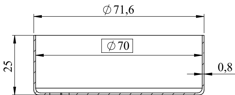
SECTION D-D
