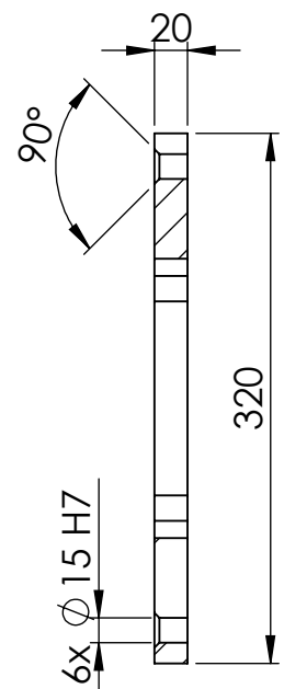
PRZEKRÓJ A-A
