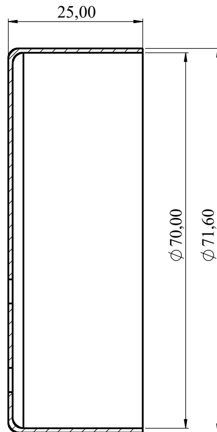
PRZEKRÓJ A-A SKALA 2 : 1
